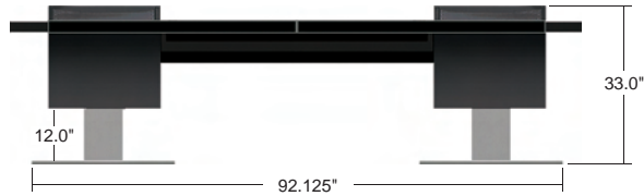
Mirage C|24 Dimensions
